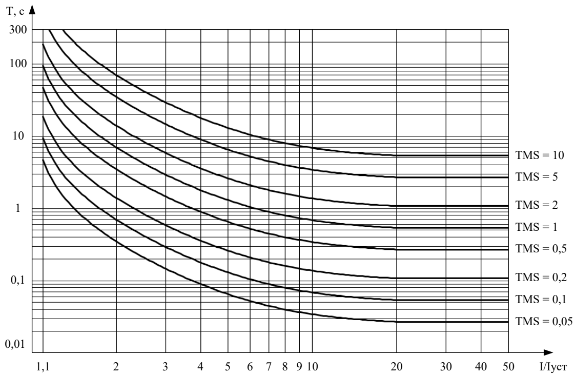
Рисунок 7 – Сильно инверсная характеристика ANSI
