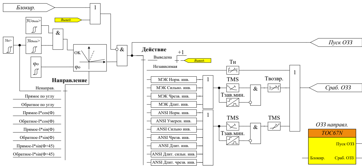
Рисунок 67 – Функциональная схема блока направленной защиты от O33 (ТНЗНП)
