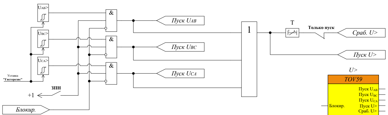
Рисунок 72 – Функциональная схема блока U>
