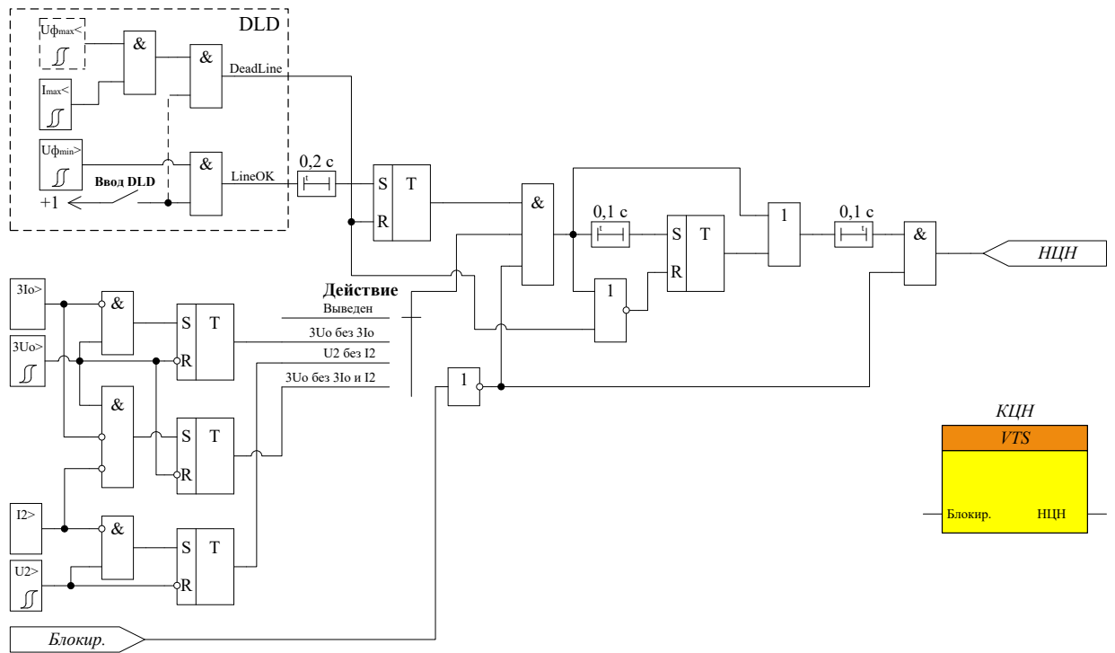
Рисунок 70 – Функциональная схема блока КЦН
