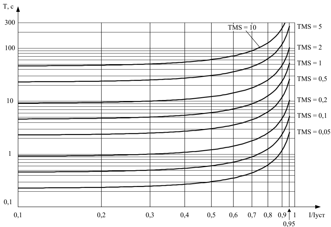
Рисунок 16 – Длительно инверсная характеристика ANSI
