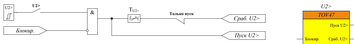
Рисунок 75 – Функциональная схема блока U2>
