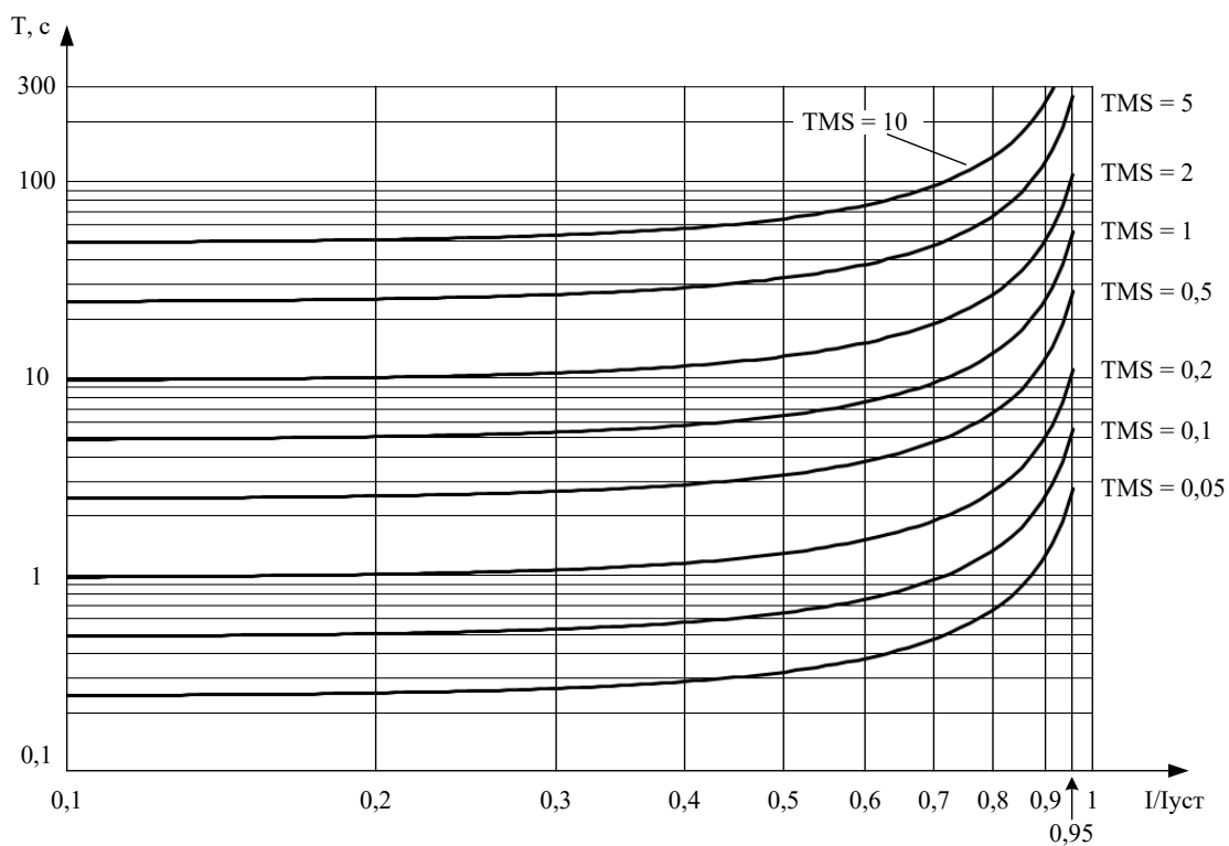
Рисунок 13 – Умеренно инверсная характеристика ANSI
