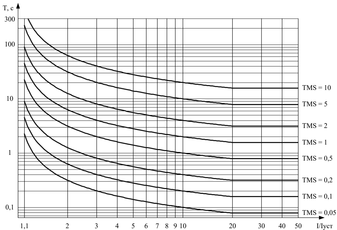
Рисунок 9 – Длительно инверсная характеристика ANSI
