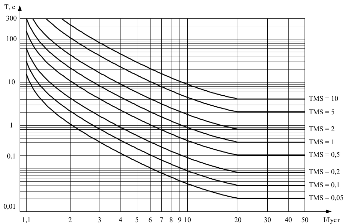
Рисунок 11 – Длительно чрезвычайно инверсная характеристика ANSI
