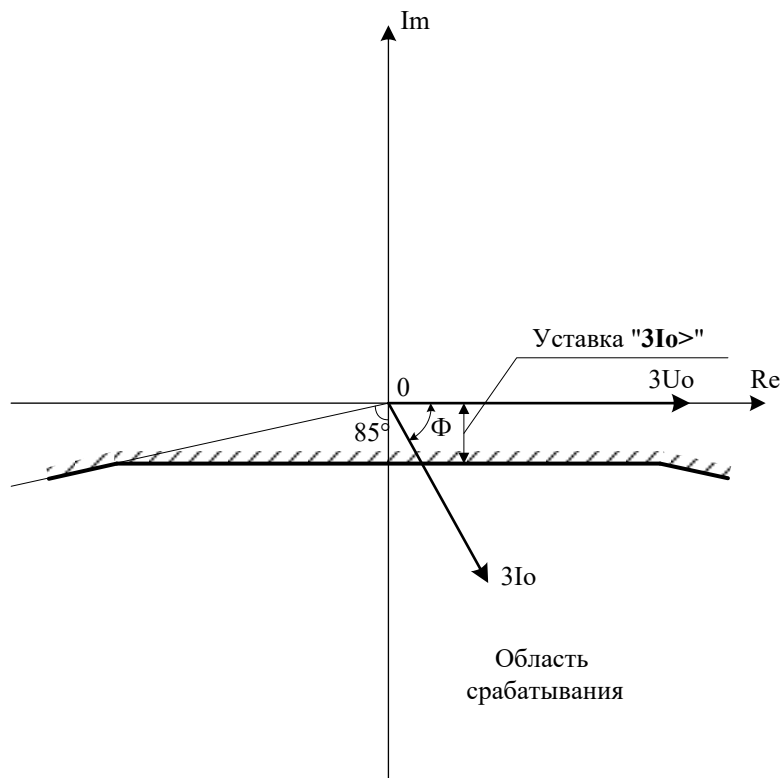
Рисунок 24 – Диаграмма направленности (Уставка "Направление": \Phi_{мч}=270; I \cdot \sin(\Phi-180) )
