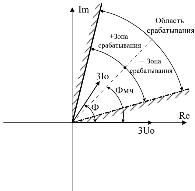
Рисунок 19 – Диаграмма направленности (Уставка "Направление": \Phi_{мч} ; \Phi_{зс} )
