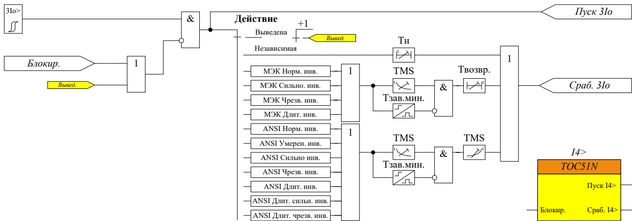
Рисунок 66 – Функциональная схема блока I4> с зависимыми характеристиками
