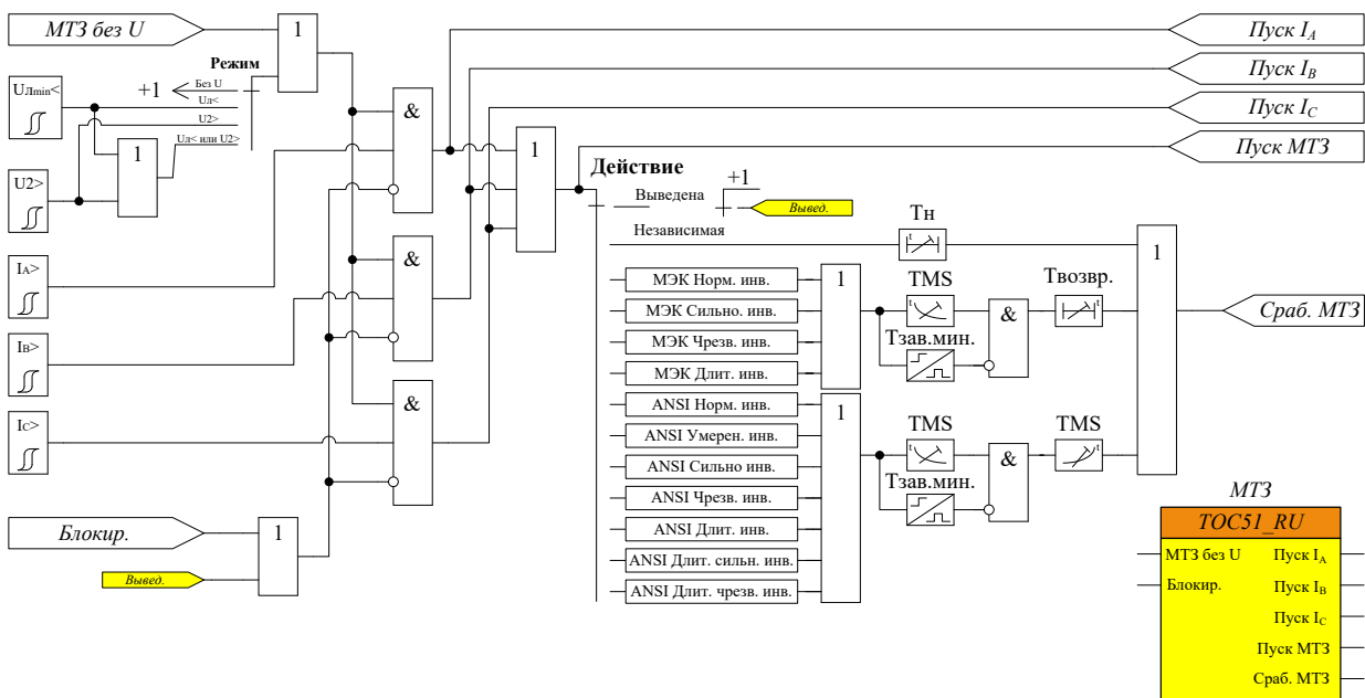
Рисунок 61 – Функциональная схема блока МТЗ с пуском по напряжению и зависимыми характеристиками
