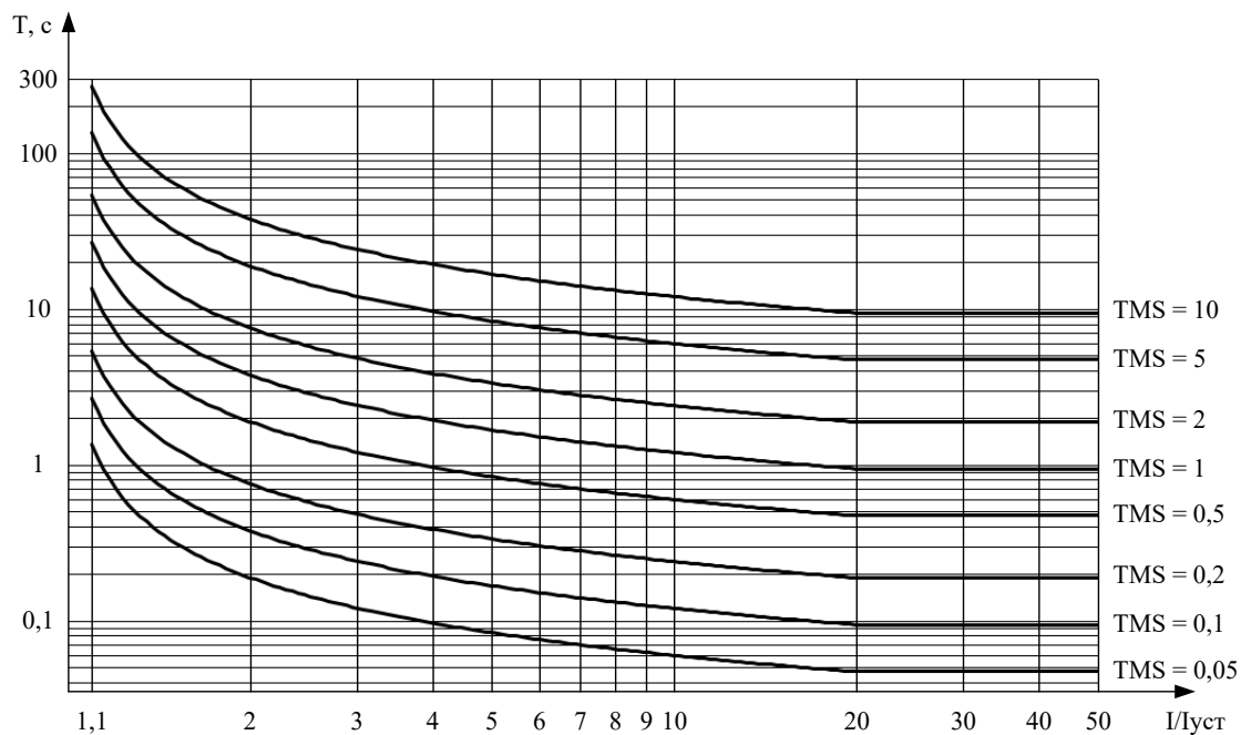
Рисунок 6 – Умеренно инверсная характеристика ANSI
