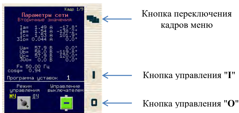
Рисунок 27 – Дисплей и кнопки на лицевой панели блока
