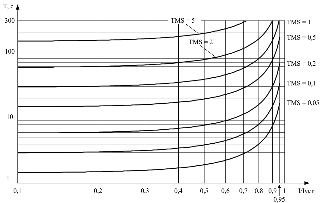
Рисунок 15 – Чрезвычайно инверсная характеристика ANSI
