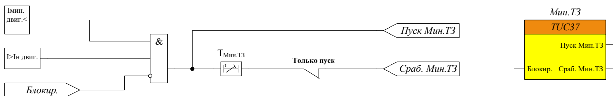
Рисунок 77 – Функциональная схема блока Мин. Т3
