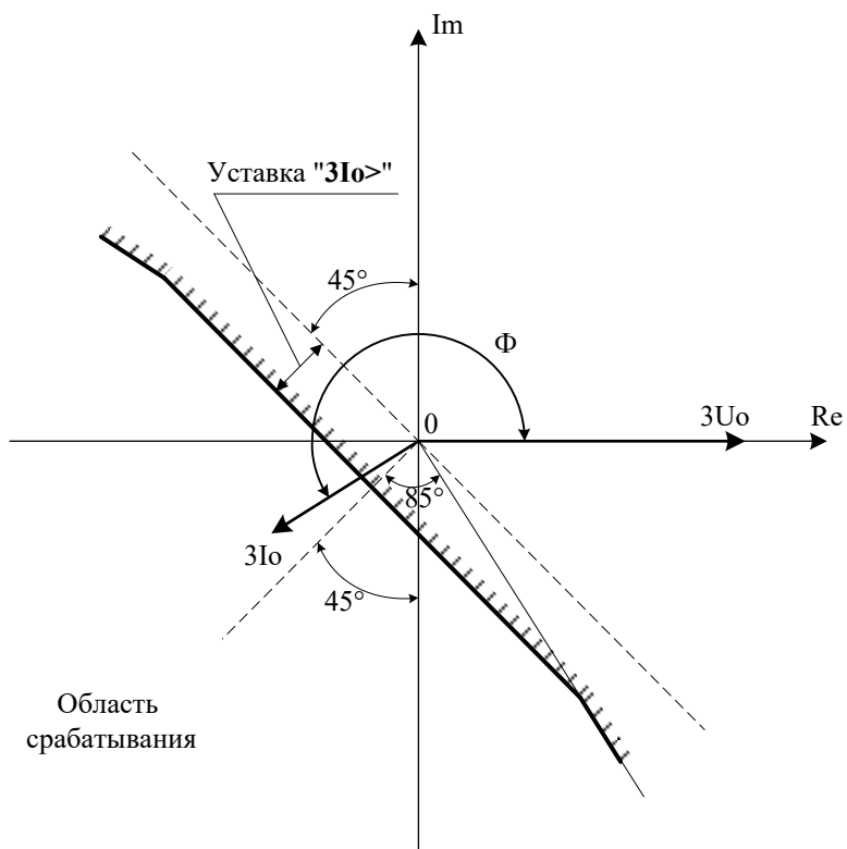
Рисунок 26 – Диаграмма направленности (Уставка "Направление": \Phi_{мч}=225; I \cdot \cos(\Phi-225) )
