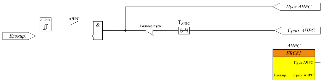
Рисунок 82 – Функциональная схема блока АЧРС
