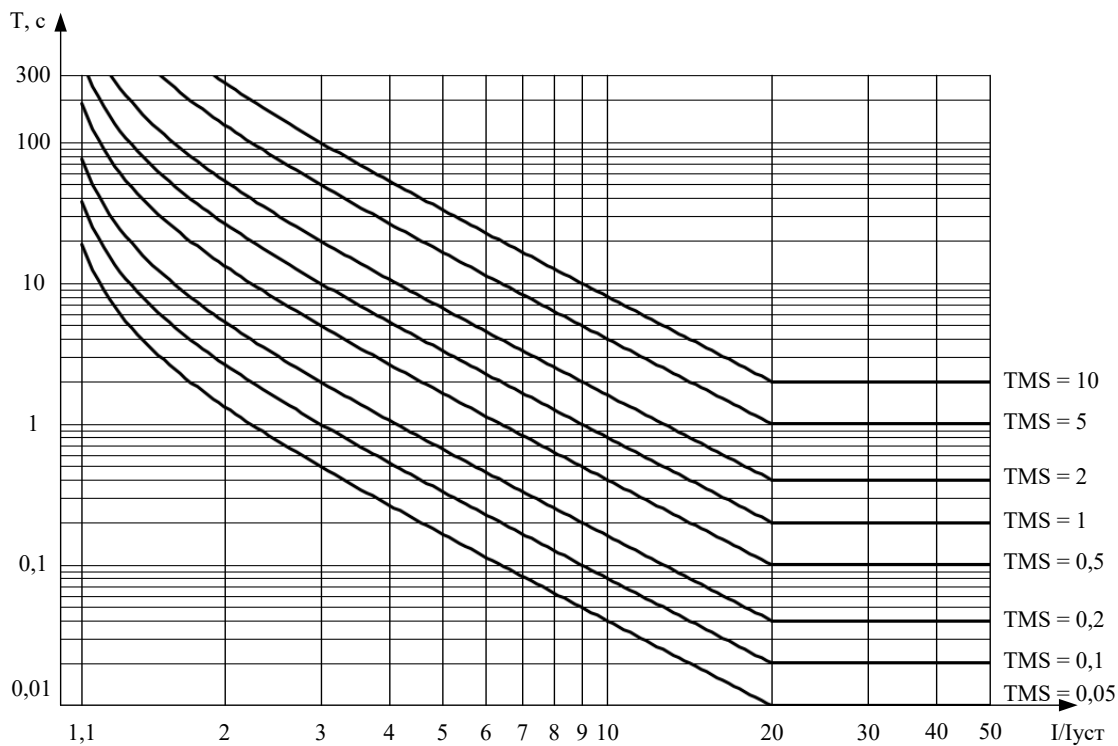
Рисунок 3 – Чрезвычайно инверсная характеристика МЭК
