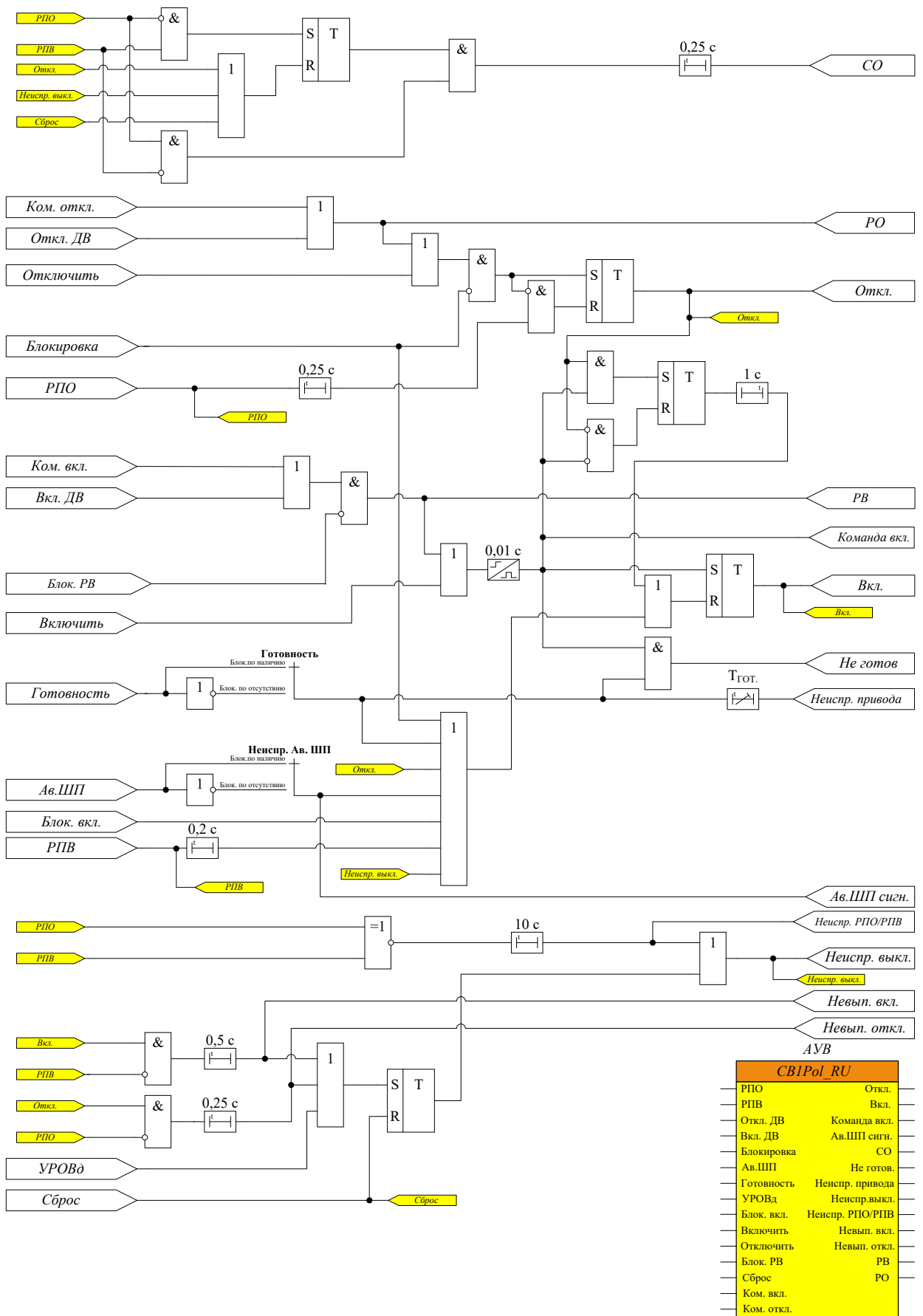
Рисунок 84 – Функциональная схема блока АУВ
