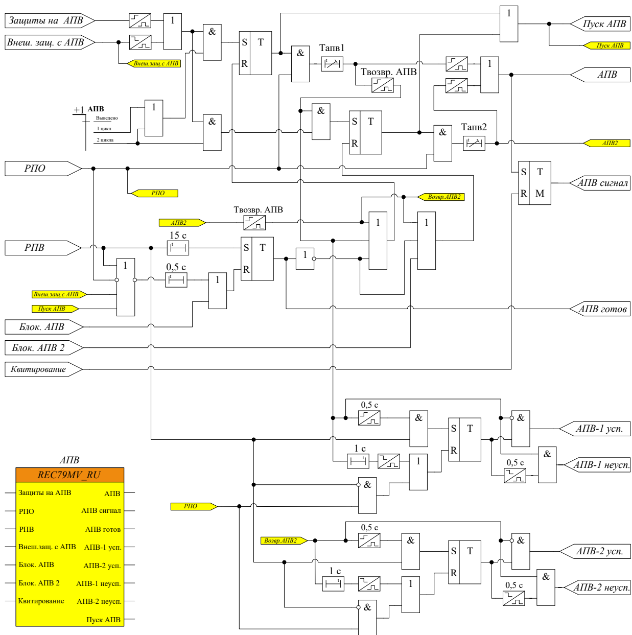
Рисунок 79 – Функциональная схема блока АПВ
