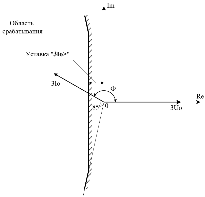
Рисунок 22 – Диаграмма направленности (Уставка "Направление": \Phi_{мч}=180; I \cdot \cos(\Phi-180) )
