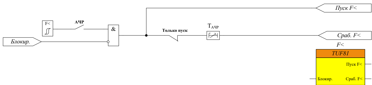
Рисунок 81 – Функциональная схема блока F<
