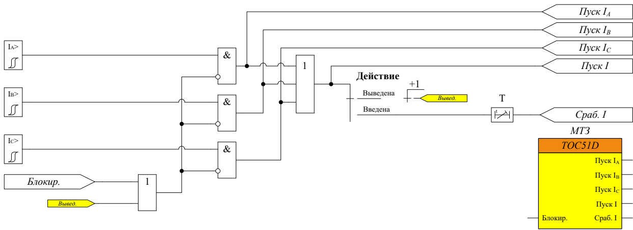
Рисунок 59 – Функциональная схема блока МТЗ
