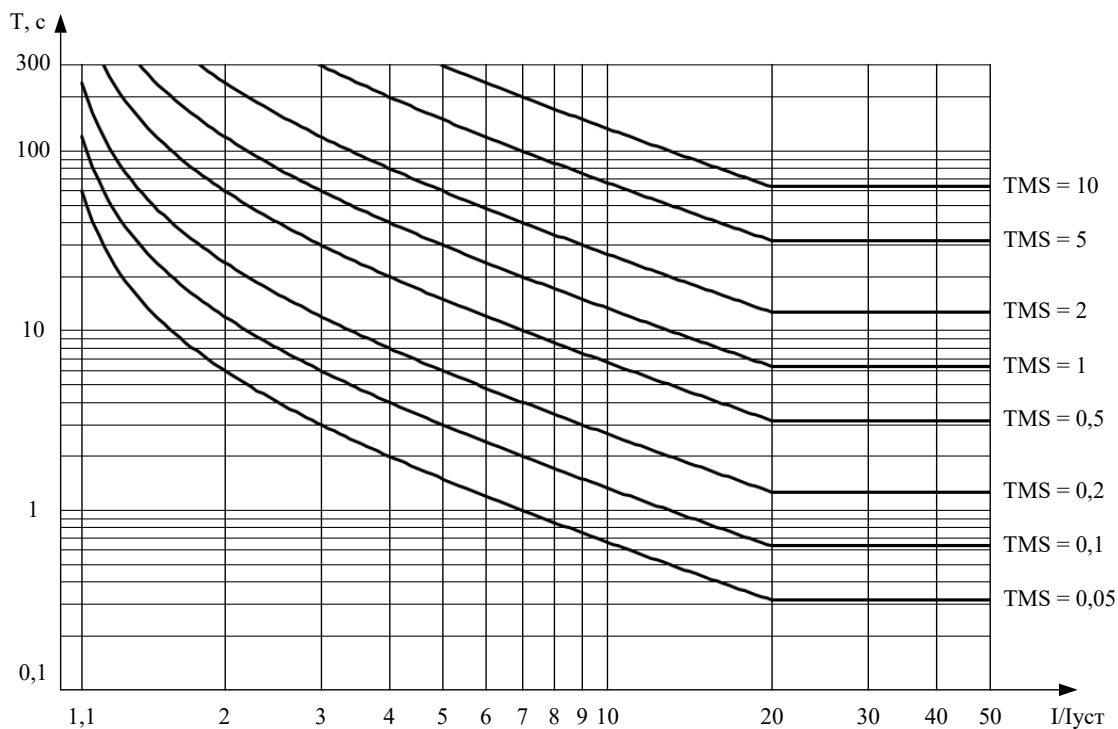
Рисунок 4 – Длительно инверсная характеристика МЭК
