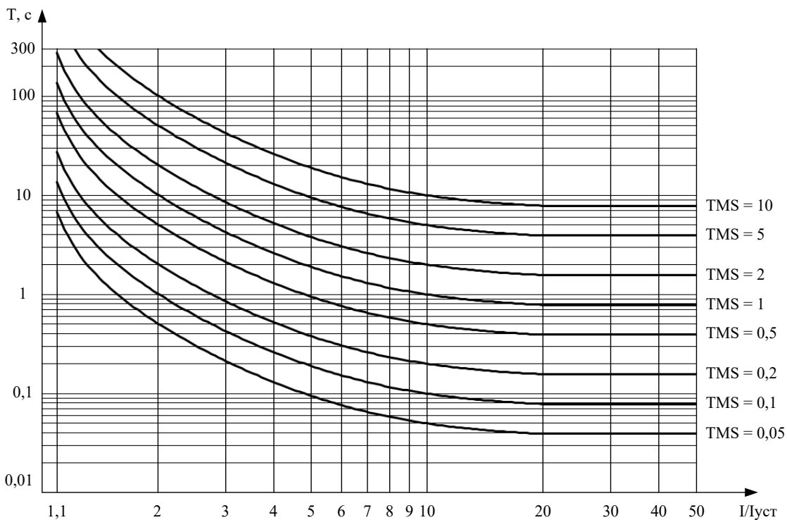
Рисунок 10 – Длительно сильно инверсная характеристика ANSI
