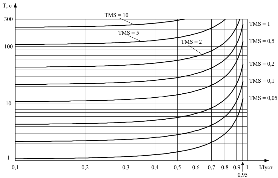
Рисунок 14 – Сильно инверсная характеристика ANSI
