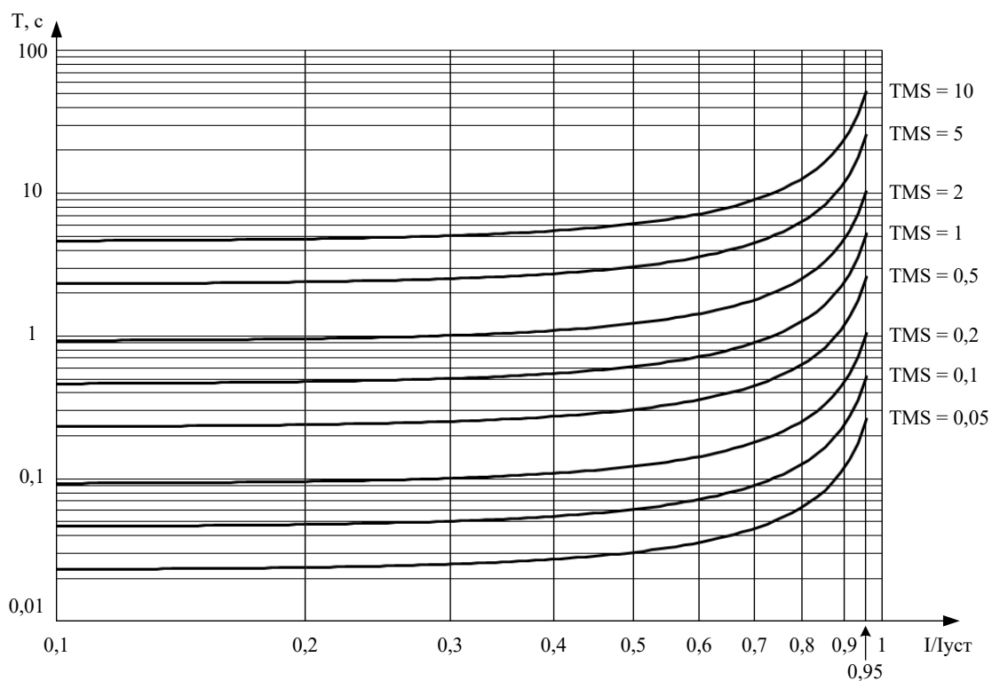
Рисунок 12 – Нормально инверсная характеристика ANSI
