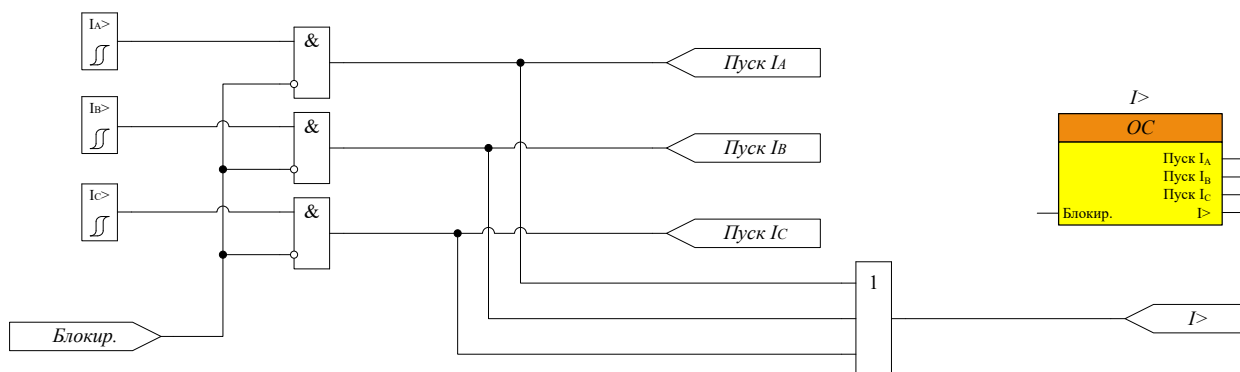
Рисунок 78 – Функциональная схема блока пускового органа УРОВ по току
