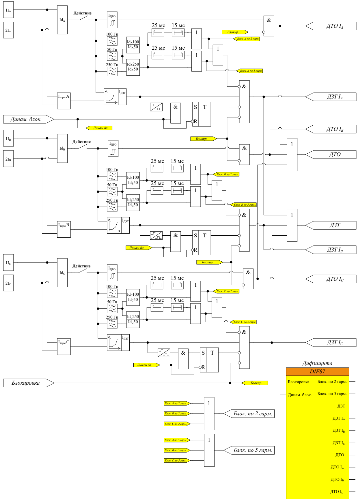
Рисунок 58 – Функциональная схема блока дифференциальной защиты
