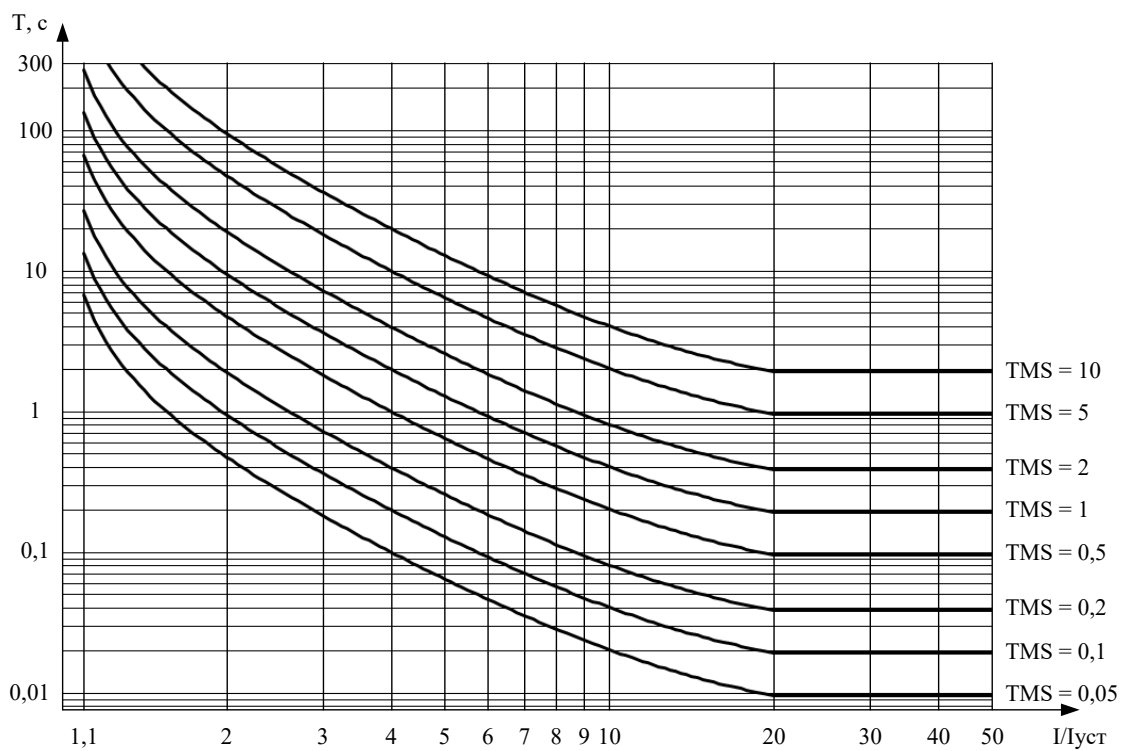
Рисунок 8 – Чрезвычайно инверсная характеристика ANSI
