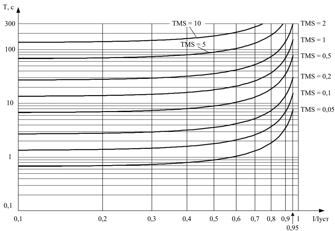
Рисунок 17 – Длительно сильно инверсная характеристика ANSI
