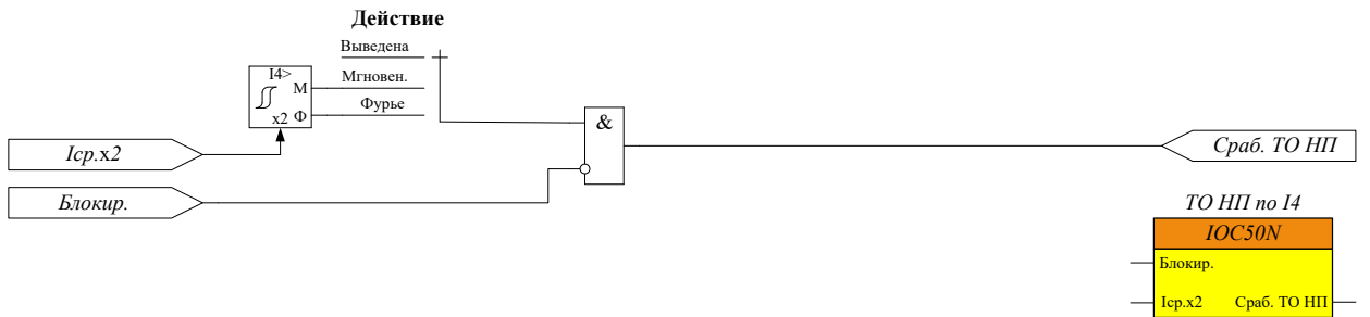
Рисунок 63 – Функциональная схема блока ТО НП по I4
