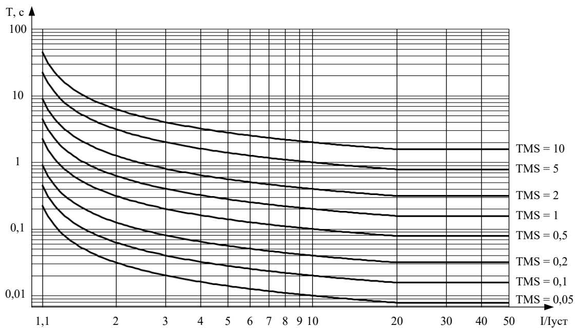
Рисунок 5 – Нормально инверсная характеристика ANSI
