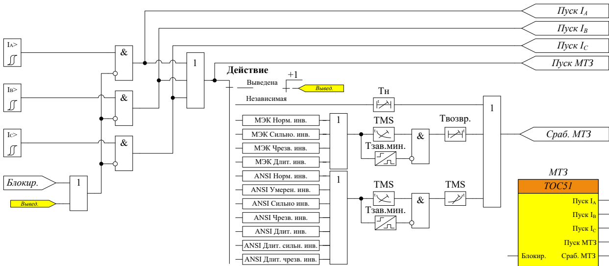
Рисунок 60 – Функциональная схема блока МТЗ с зависимыми характеристиками
