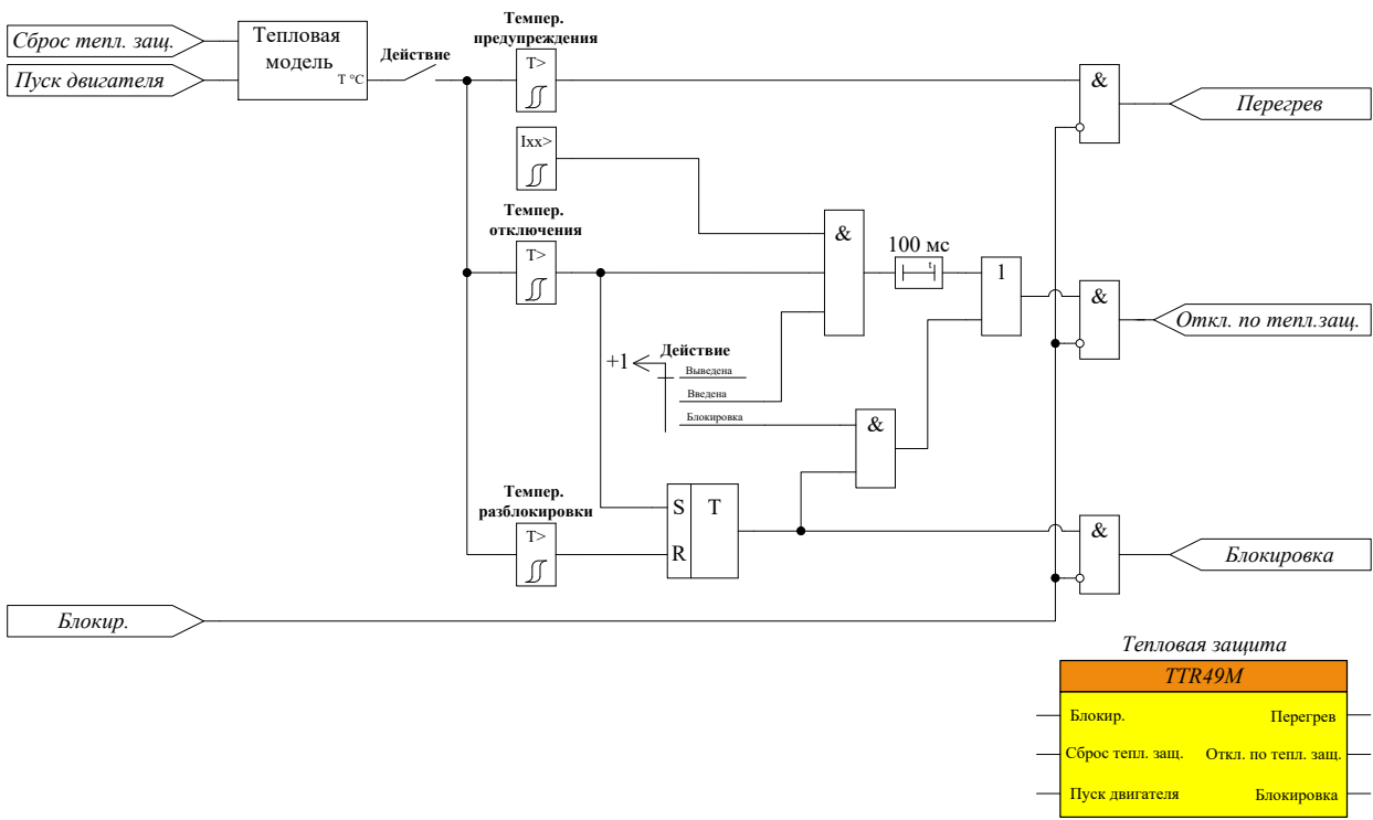
Рисунок 85 – Функциональная схема блока тепловой защиты электродвигателя
