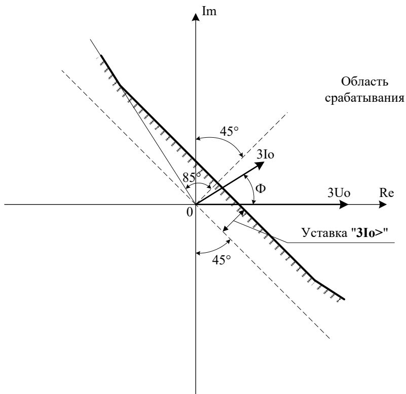
Рисунок 25 – Диаграмма направленности (Уставка "Направление": \Phi_{мч}=45; I \cdot \cos(\Phi-45) )
