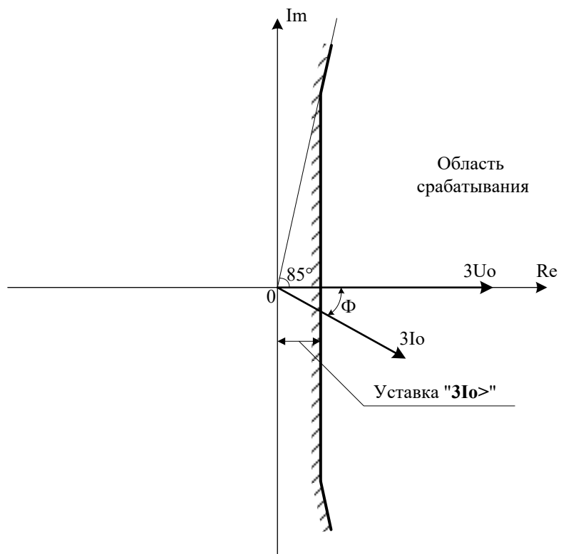
Рисунок 21 – Диаграмма направленности (Уставка "Направление": \Phi_{мч}=0; I \cdot \cos \Phi )
