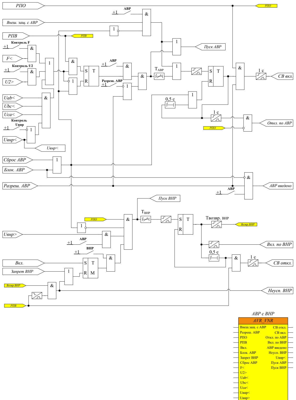
Рисунок 80 – Функциональная схема блока автоматического включения резерва с восстановлением нормального режима
