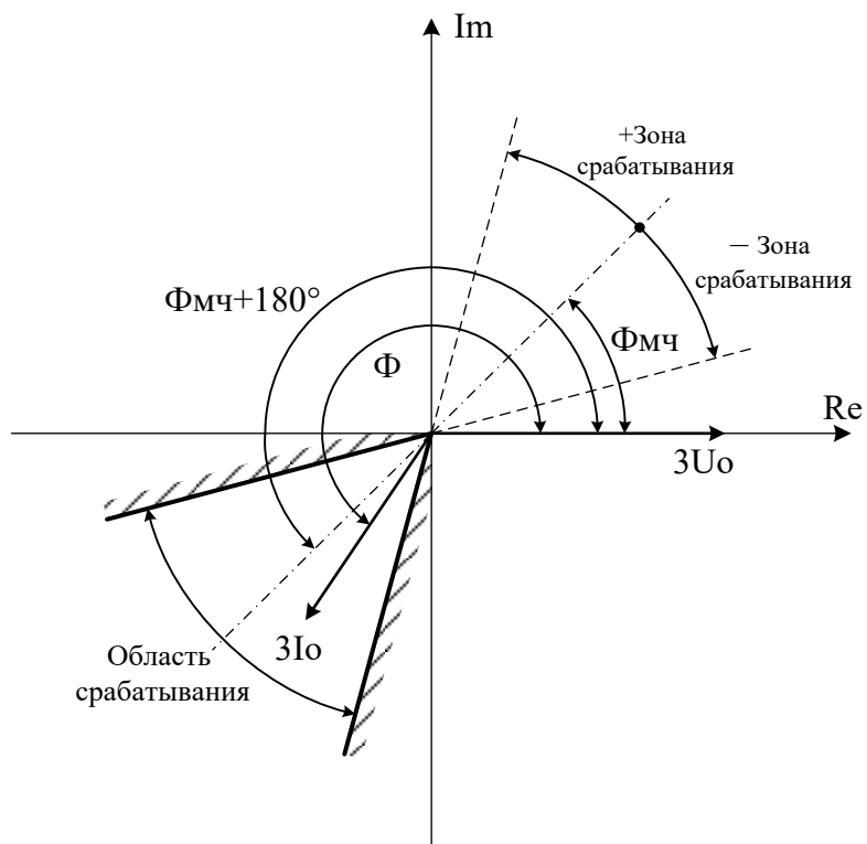
Рисунок 20 – Диаграмма направленности (Уставка "Направление": \Phi_{мч+180} ; \Phi_{зс} )
