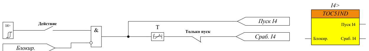
Рисунок 65 – Функциональная схема блока по I4>
