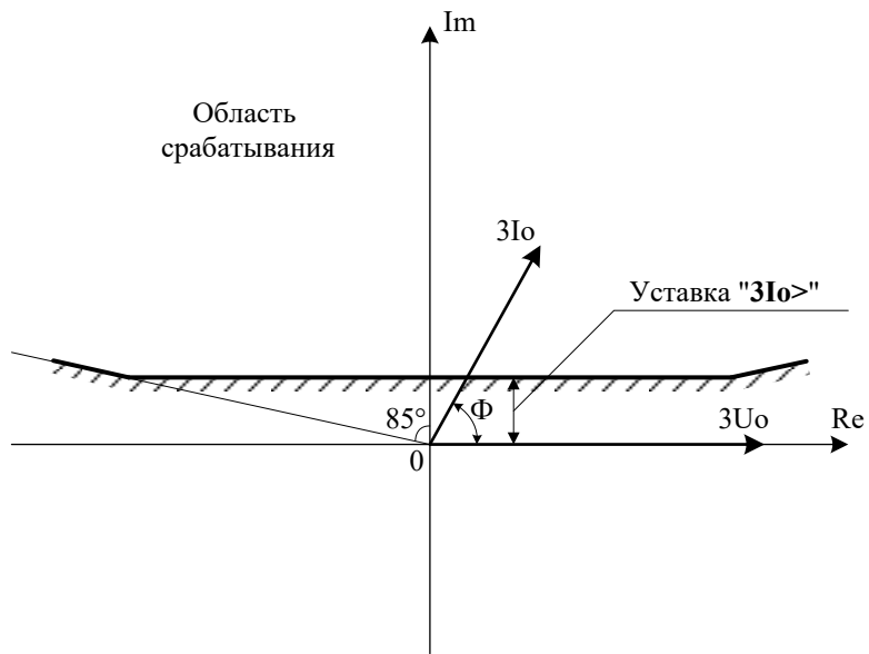
Рисунок 23 – Диаграмма направленности (Уставка "Направление": \Phi_{мч}=90; I \cdot \sin \Phi )
