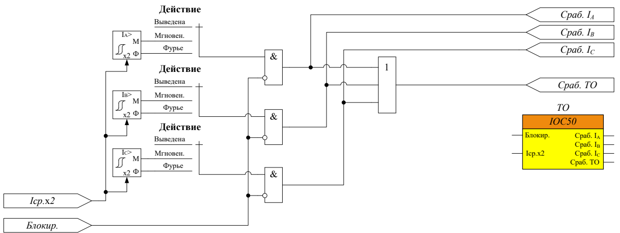
Рисунок 62 – Функциональная схема блока ТО
