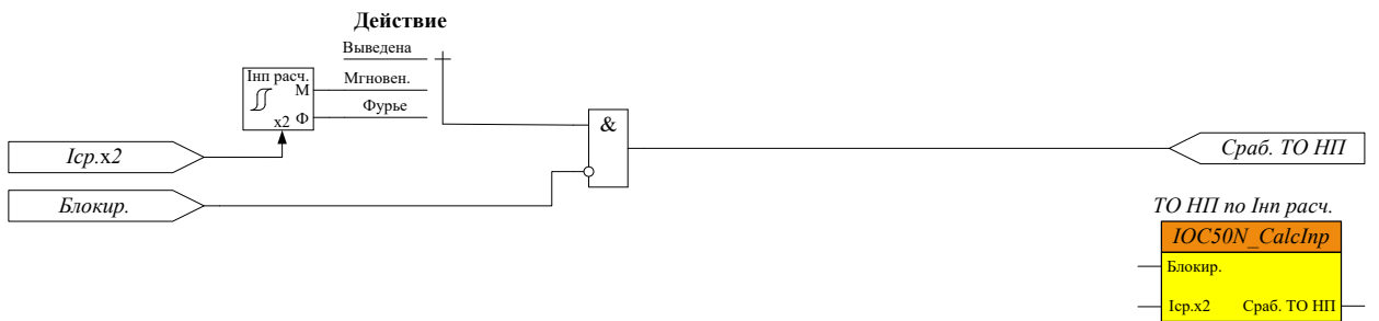
Рисунок 64 – Функциональная схема блока ТО НП по Инп расчётному
