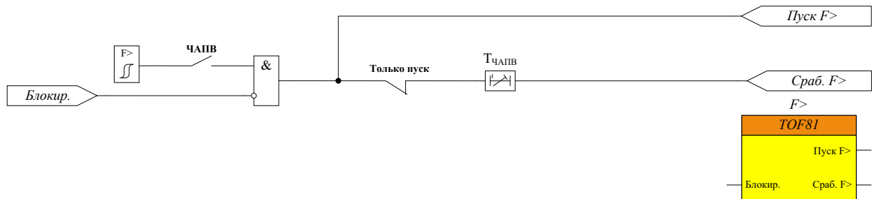
Рисунок 83 – Функциональная схема блока F>
