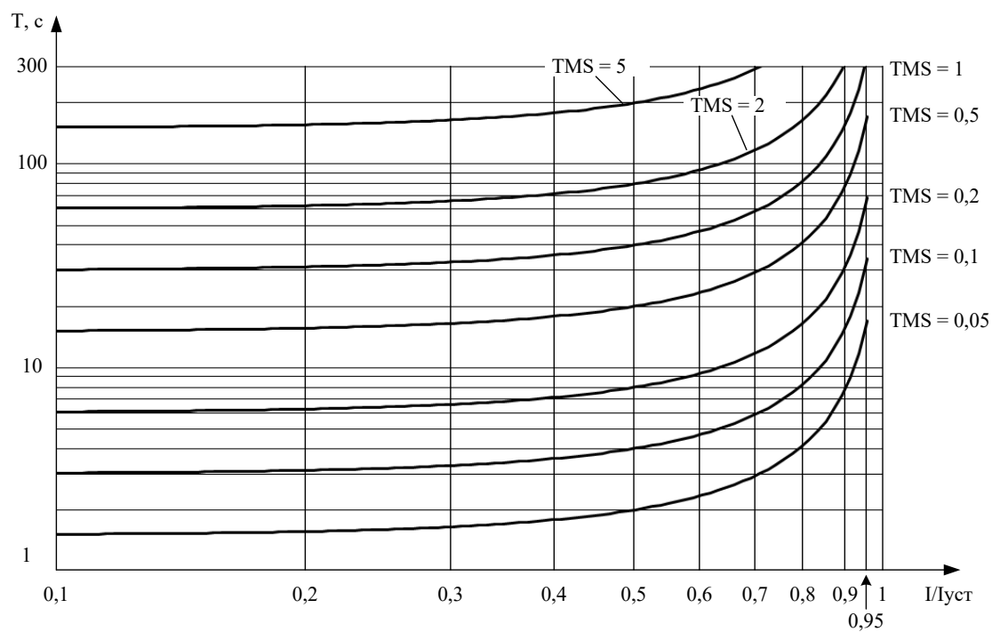
Рисунок 18 – Длительно чрезвычайно инверсная характеристика ANSI
