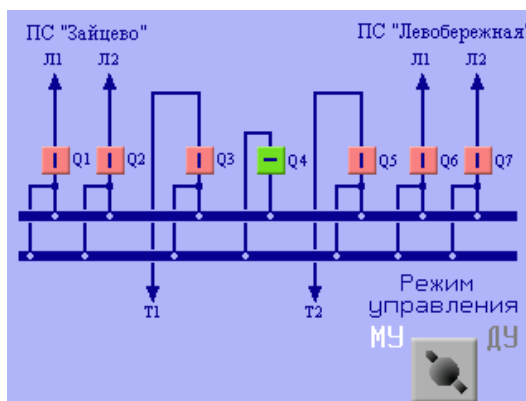
Рисунок 28 – Кадр "Однолинейная схема"
