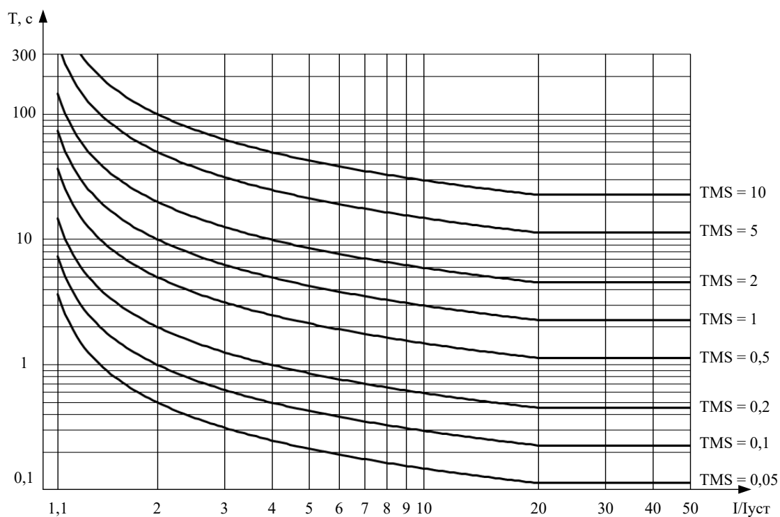
Рисунок 1 – Нормально инверсная характеристика МЭК
