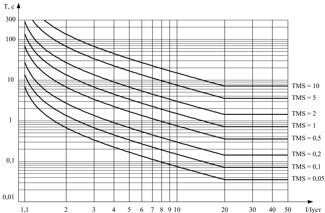
Рисунок 2 – Сильно инверсная характеристика МЭК
