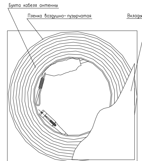
Рисунок 6а – Схема укладки кабеля антенны приемника
